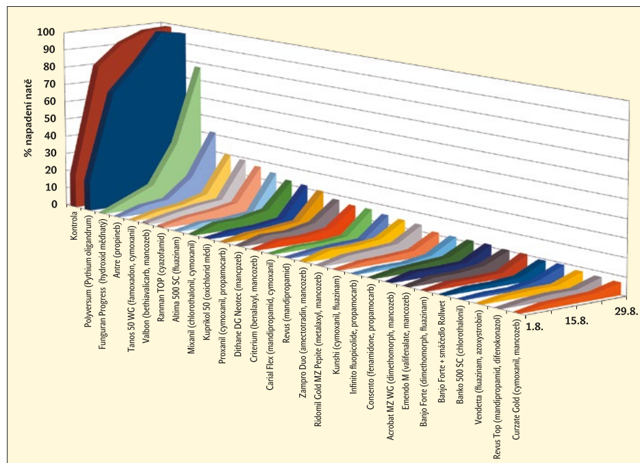
Graf 4: Vývoj plísňe bramboru v nati v roce 2016 (Valečov, odrůda Ditta, výběr fungicidů)
