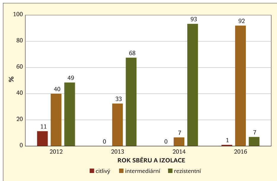
Graf 9: Procentuální zastoupení citlivých, intermediárních a rezistentních izolátů k propamokarb-hydrochloridu v letech 2012–2014 a 2016
