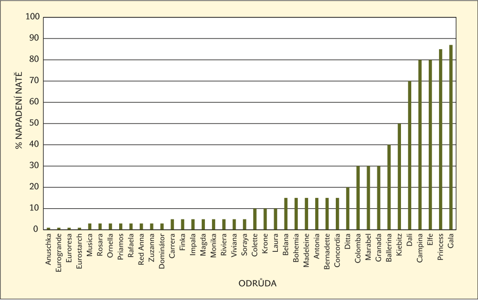
Graf 3: Procento napadení natě plísní bramboru u vybraných odrůd k 22. 8. 2016 (ošetřeno proti plísni bramboru, výběr odrůd s plochou nad 10 ha množení v ČR)
