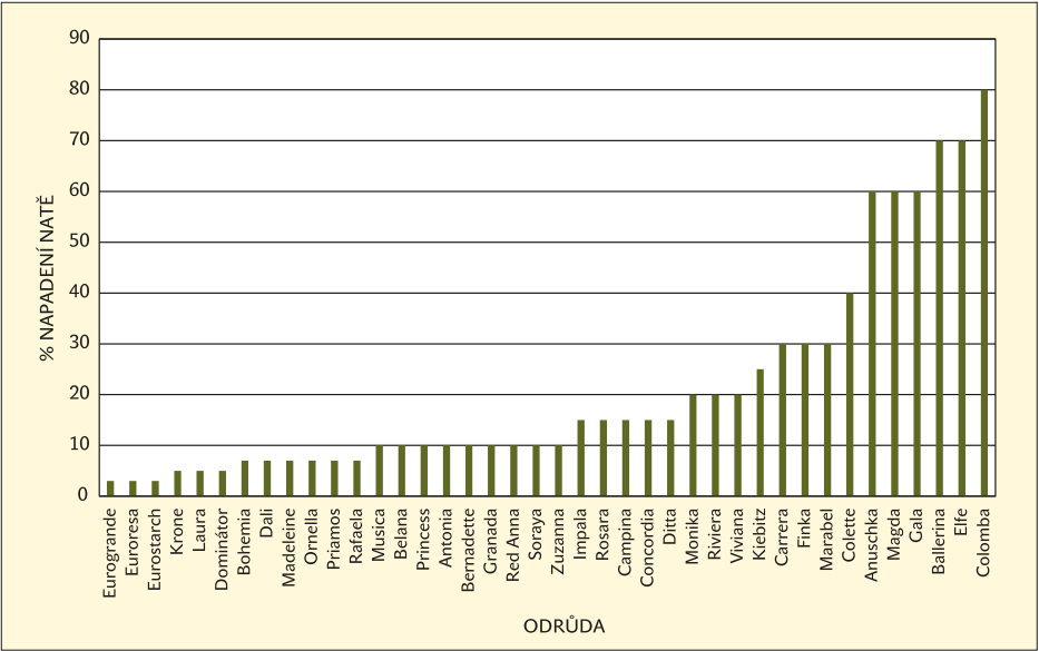
Graf 2: Procento napadení natě plísní bramboru u vybraných odrůd k 1. 8. 2016 (Valečov, neošetřeno proti plísni bramboru, výběr odrůd s plochou nad 10 ha množení v ČR)
