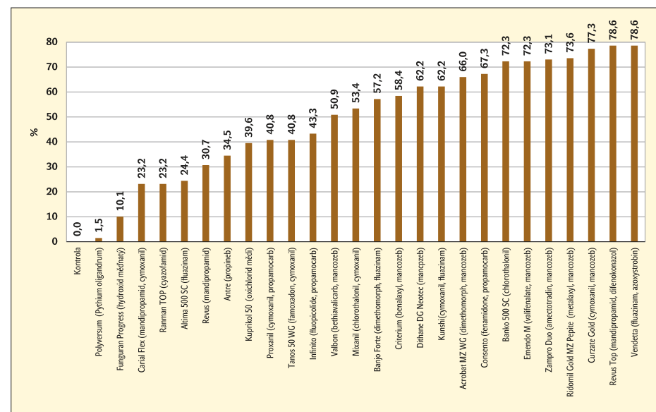
Graf 5: Procento účinnosti (Abbott) vybraných fungicidů na směšnou infekci plísní bramboru a alternariiových skvrnitostí k 6. 9. 2016 (Valečov, odrůda Ditta)
