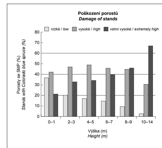
Obr. 13: Závislost poškození SMP na průměrné výšce porostu Fig. 13: A dependence of damage of Colorado blue spruce stands on tree height of stand
