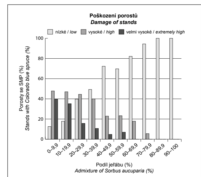
Obr. 14: Závislost poškození SMP na podílu JR Fig. 14: A dependence of damage of Colorado blue spruce stands on the admixture of Sorbus aucuparia in stands
