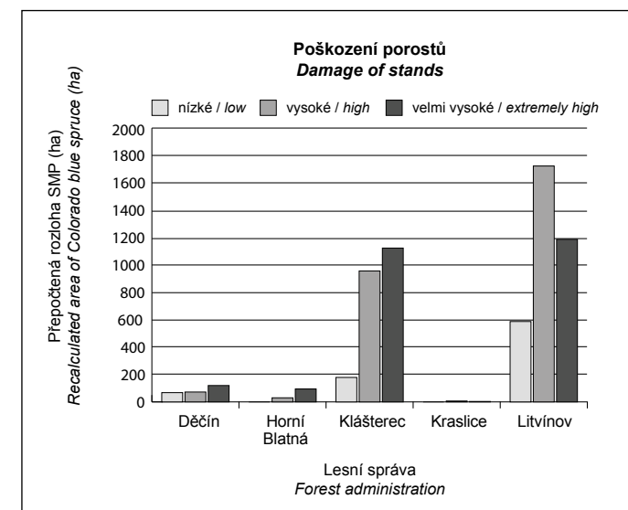
Obr. 15: Přepočtená rozloha porostů SMP (dle ÚHÚL) v jednotlivých kategoriích poškození dle LS Fig. 15: The recalculated area of Colorado blue spruce stands (according to the UHÚL) in the individual damage categories according to particular forest administrations
