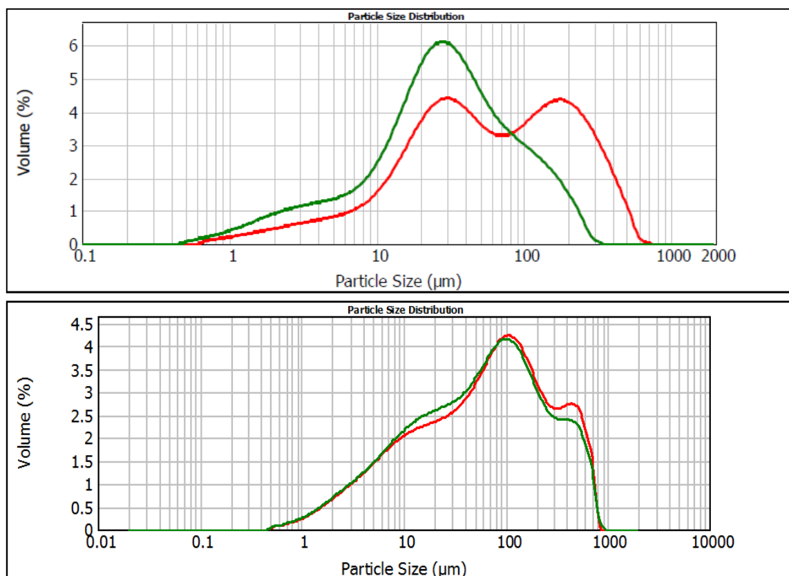
Obr. 20: Distribuce velikosti částic mezi prolisy ze surového lněného oleje před deskovou filtraceí (horní obrázek) a lisovaného řepkového oleji izolovaném v závodu s kapacitou 1500 t/den před průmyslovým usazováním a filtraceí na Amafiltru (spodní obrázek)
