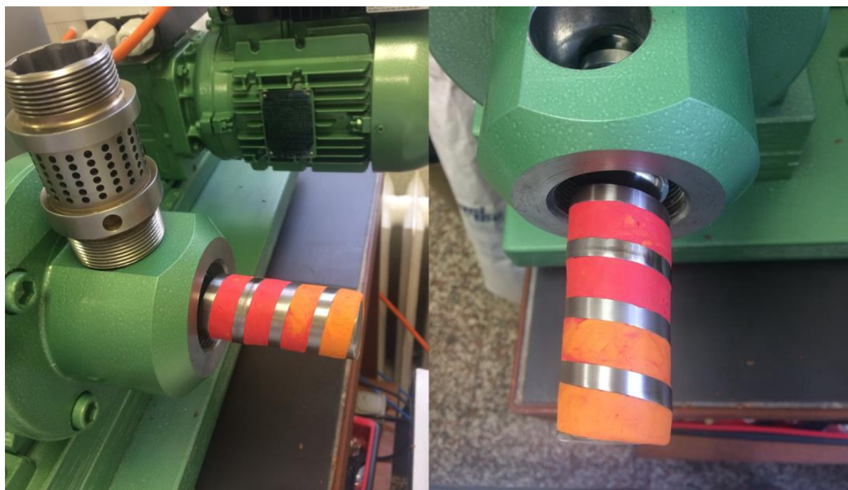
Obr. 10: Stanovení objemu závitu a objemu cedáku (přístroji Komet CA59G, IBG Monforts Oekotec GmbH & Co.KG, Germany) schematicky (Foto: J. Kyselka)
