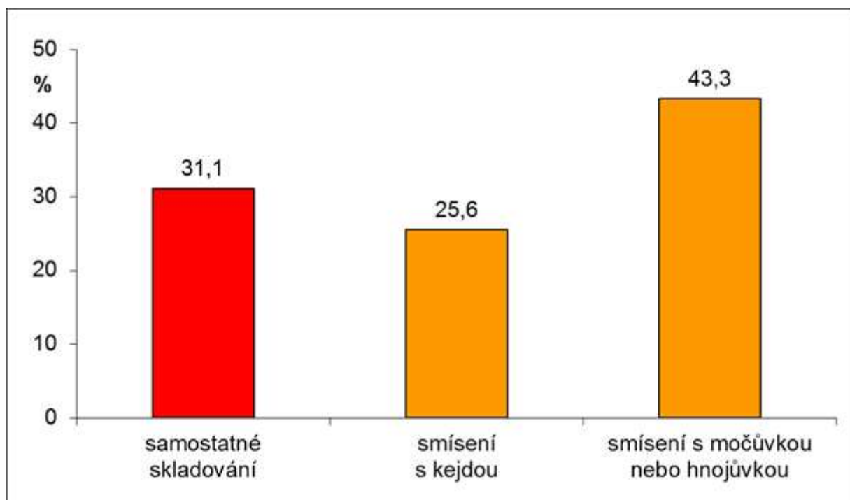
Graf 6: Způsob nakládání s technologickými vodami v závodech
