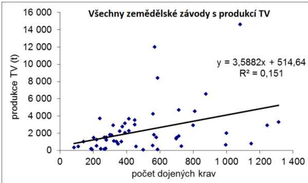
Graf 7: Vztah mezi počtem dojených krav a celkovou produkcí technologických vod (TV) v zemědělských závodech
