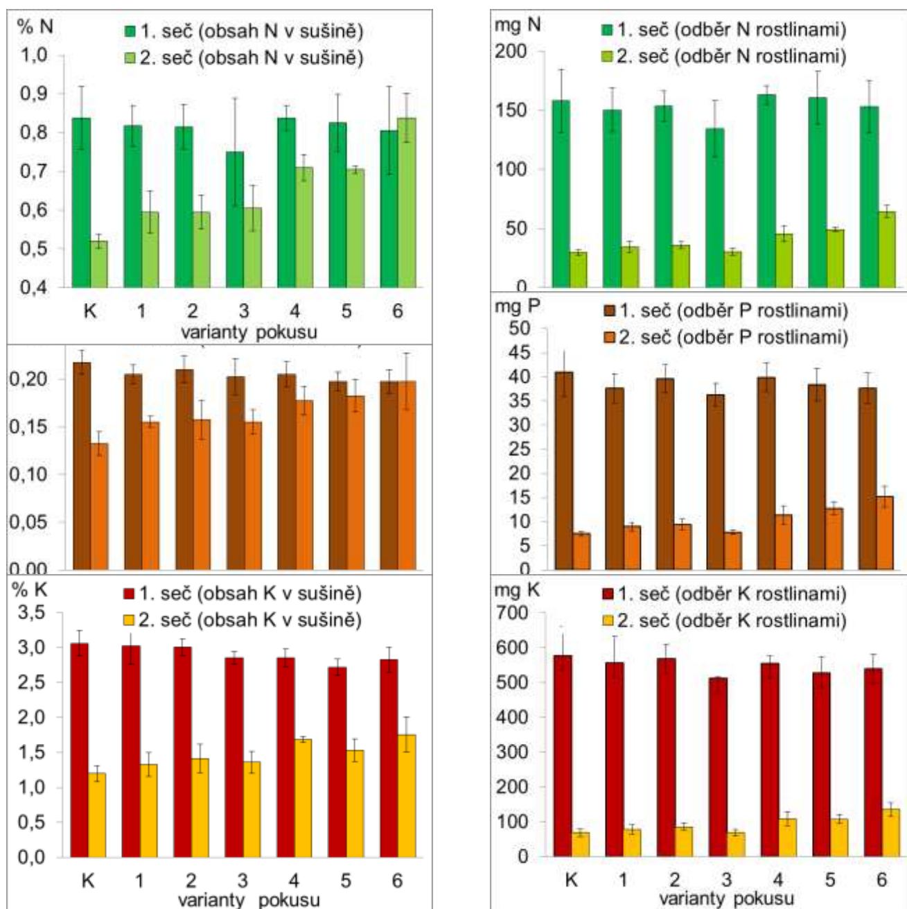
Graf 10: Obsah a odběr živin rostlinami jílku vytrvalého v nádobovém pokusu (obsah živin v % v sušině, odběr živin v mg na pokusnou nádobu)
